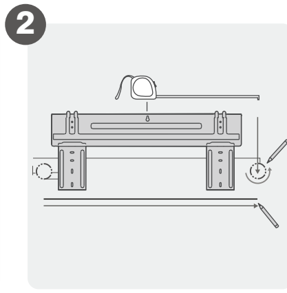
Fest monteringsplaten
