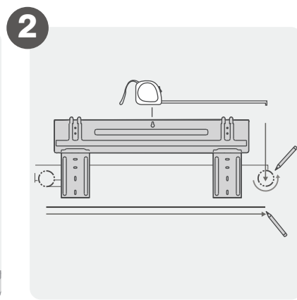
Fastgør monteringspladen
