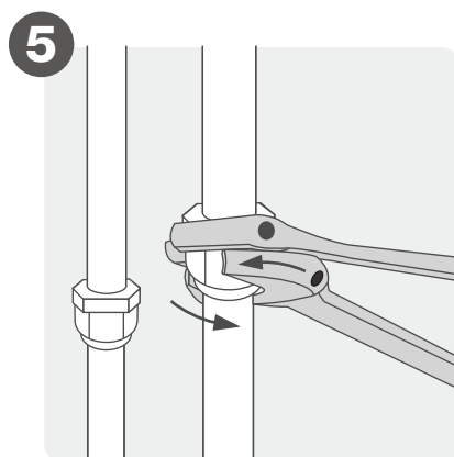
Anslut rören
