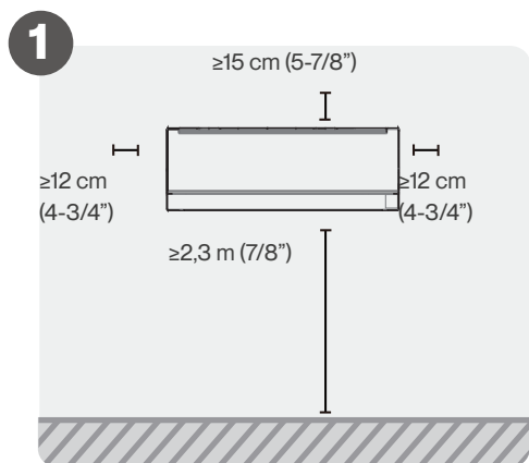
Vælg installationsplacering
