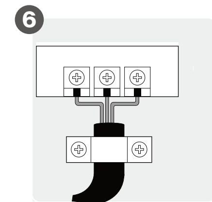
Tilslut ledninger
